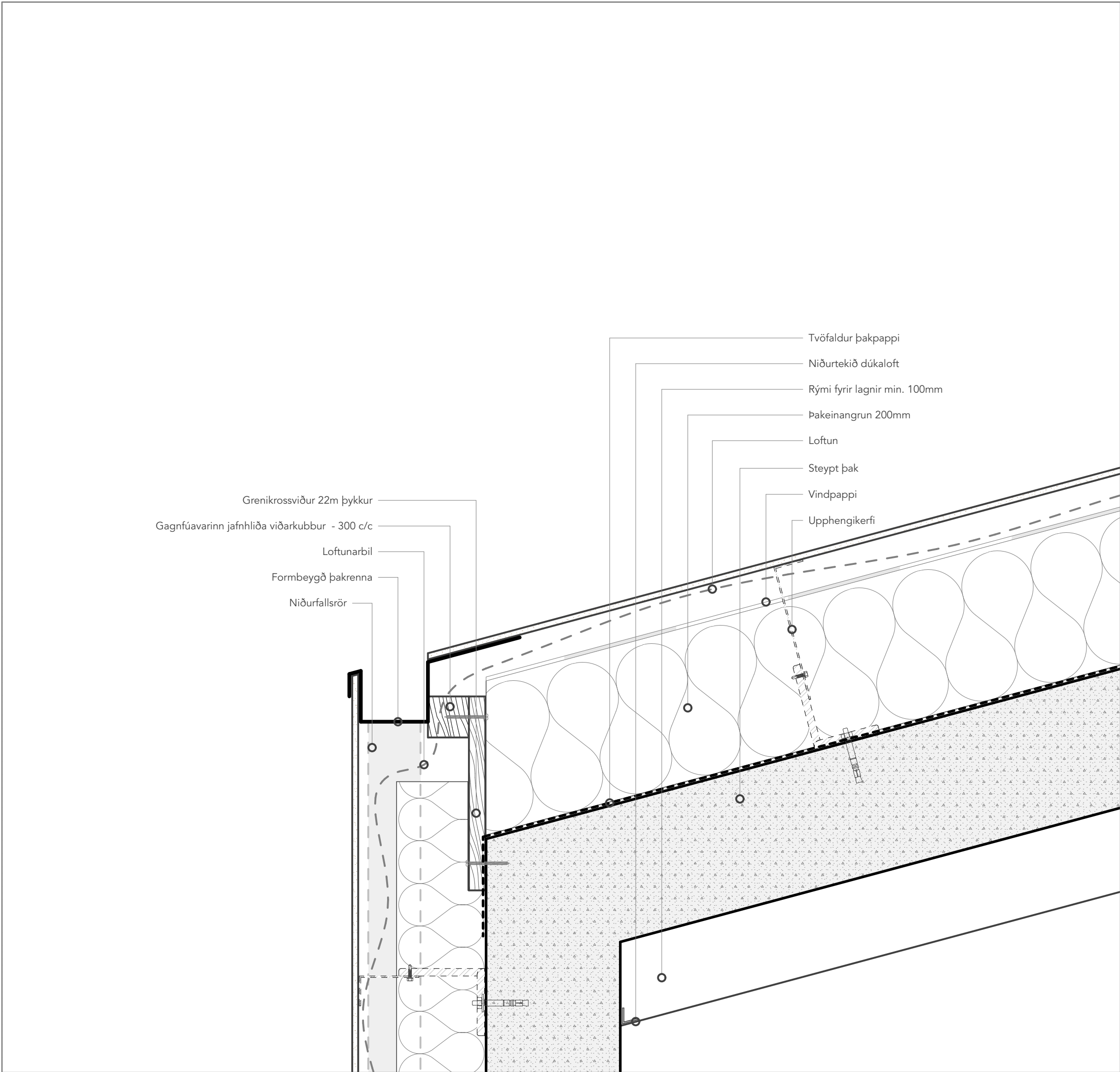
D-1 Einhalla þak - lægsti punktur 1:5
