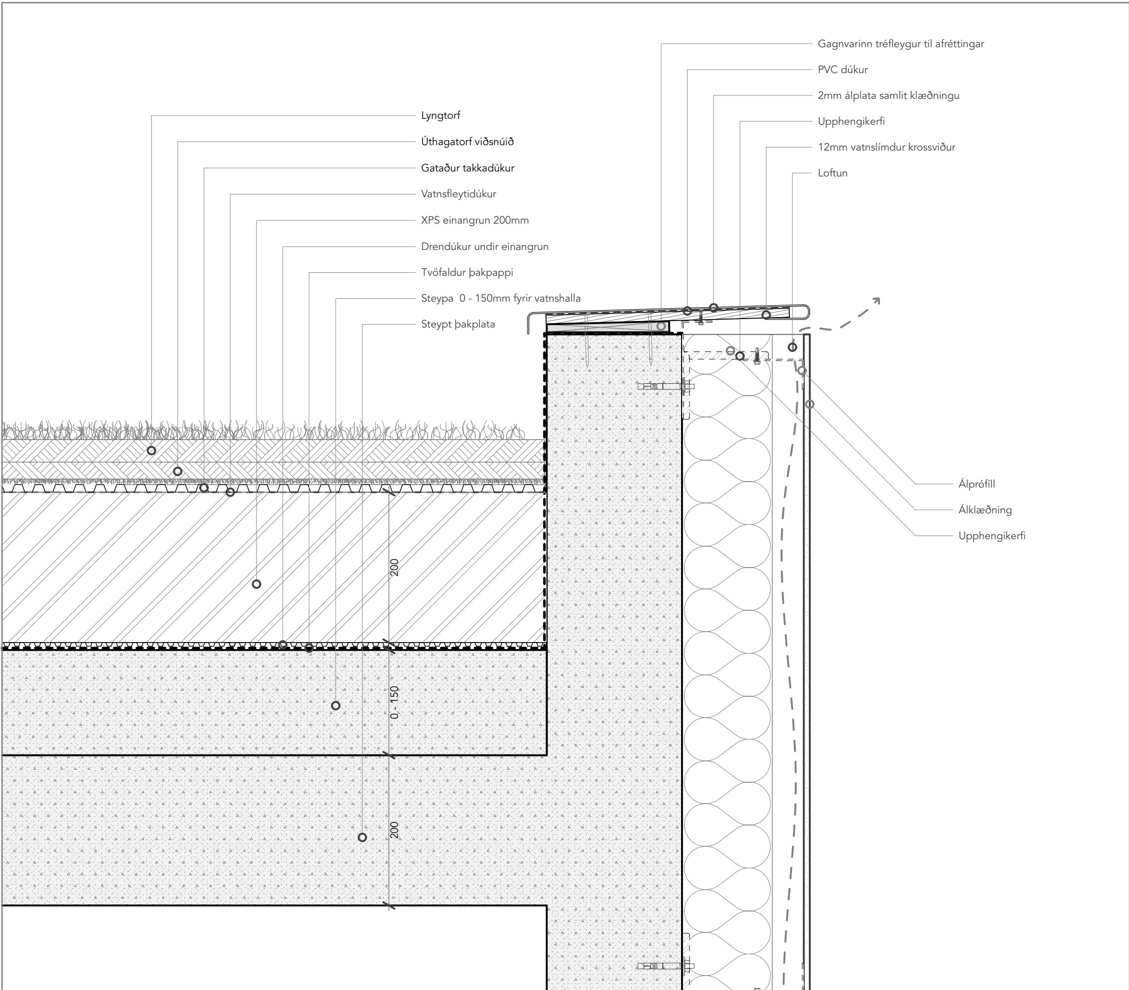
D-3 Flatt þak við þakkant 1:5
