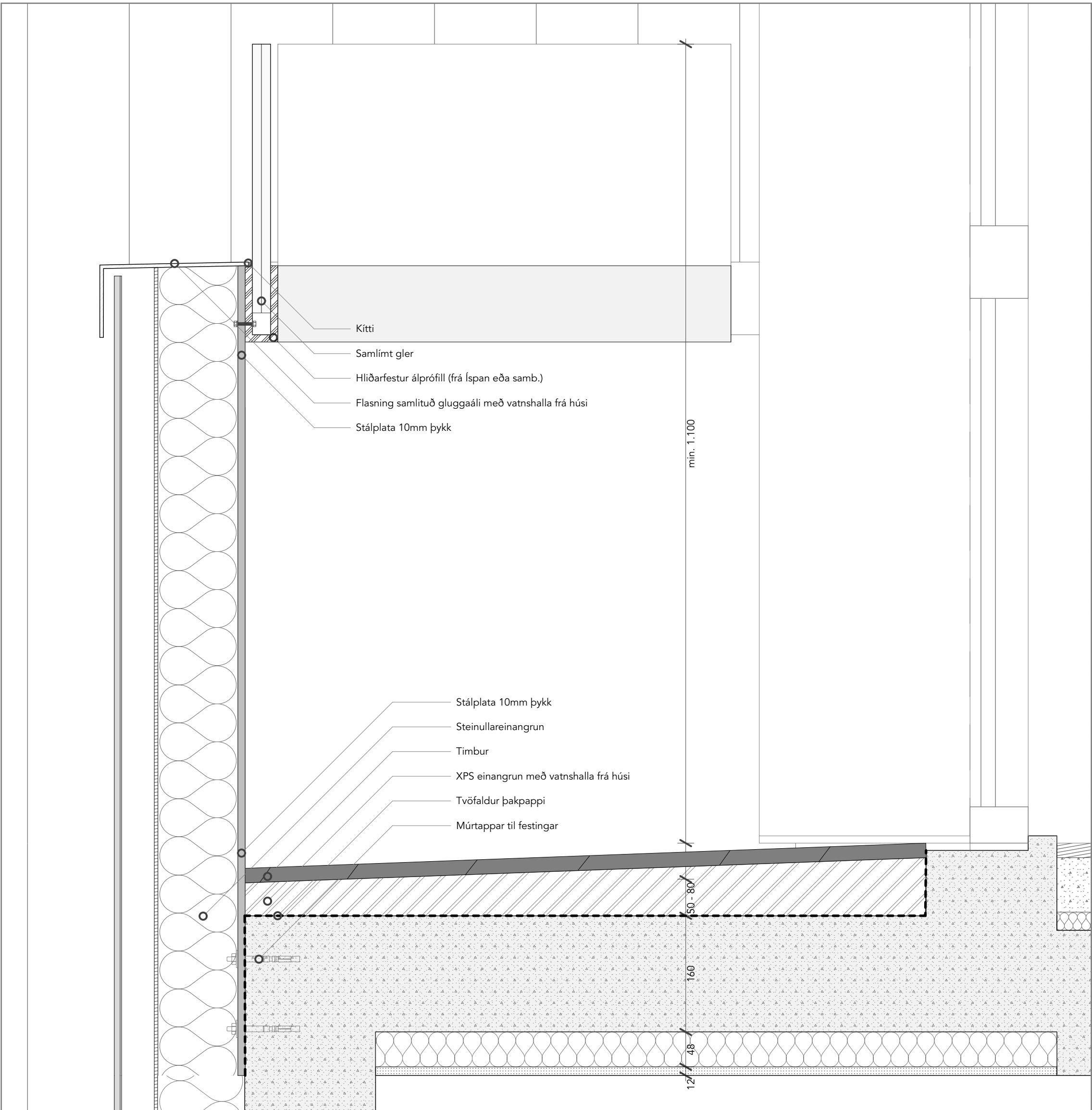
D-8 Svalir og svalahandrið 1:5
