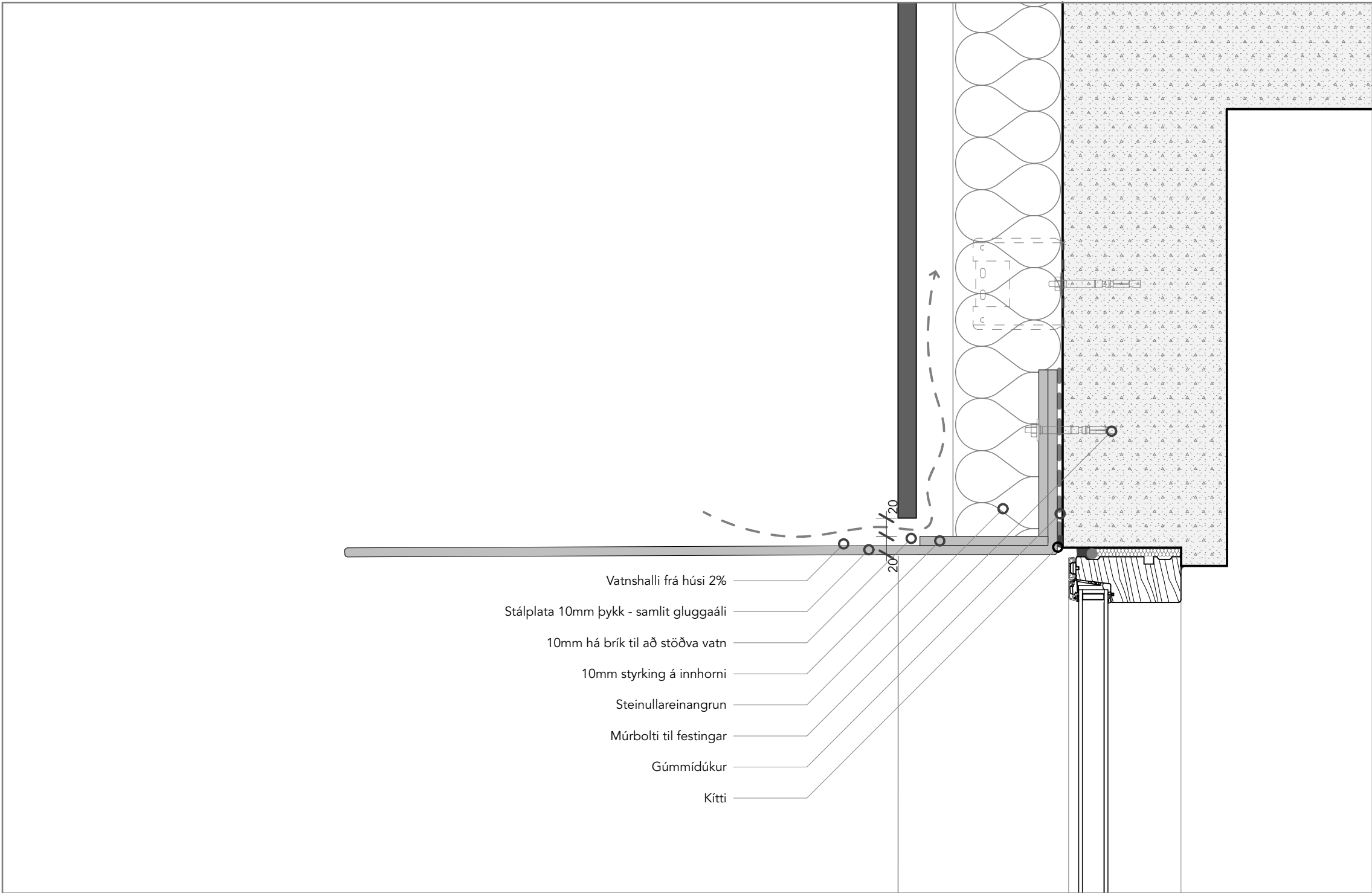
D-5 Skyggni yfir aukaíbúð 1:5
