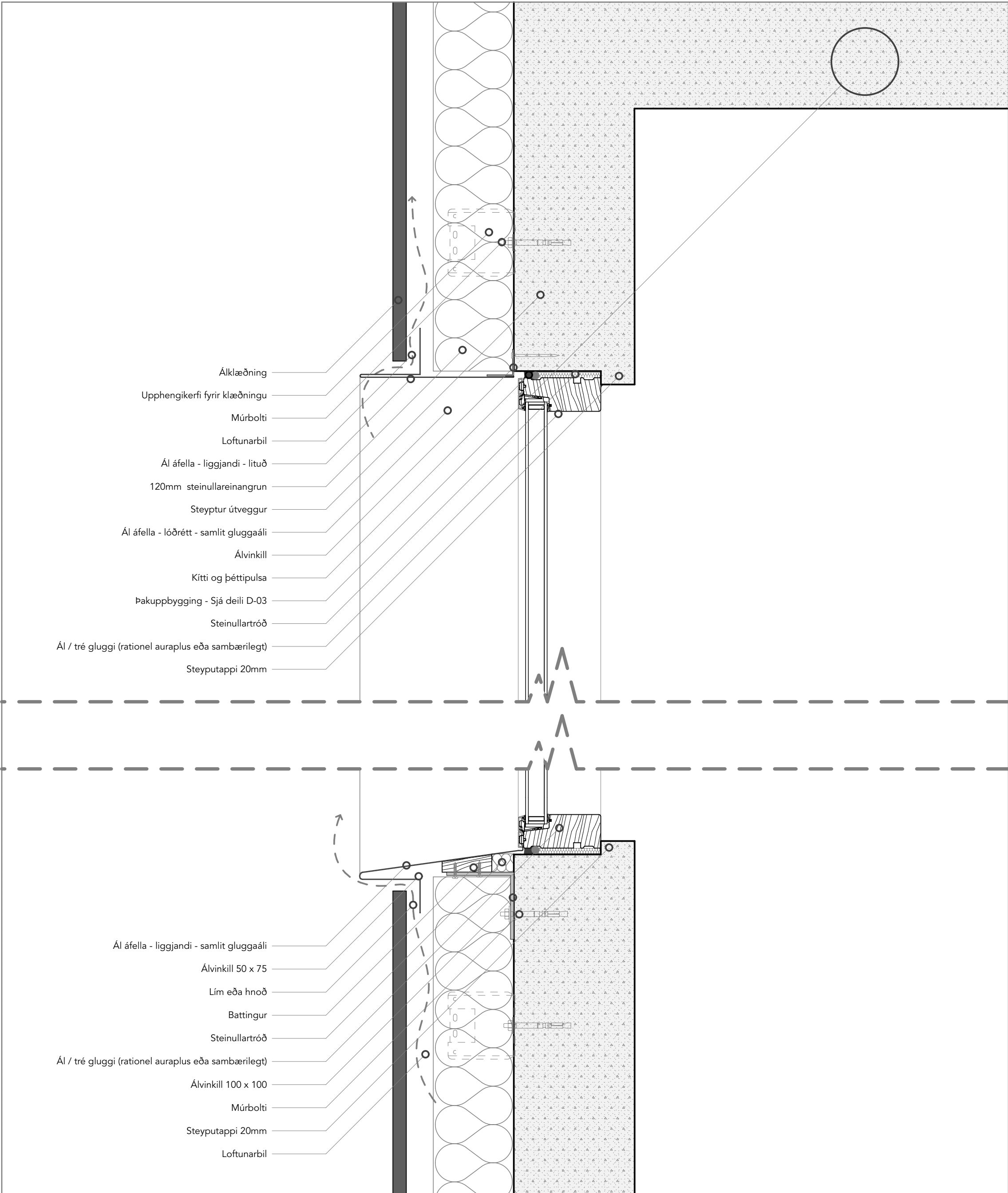
D-7 Gluggafrágangur 1:5
