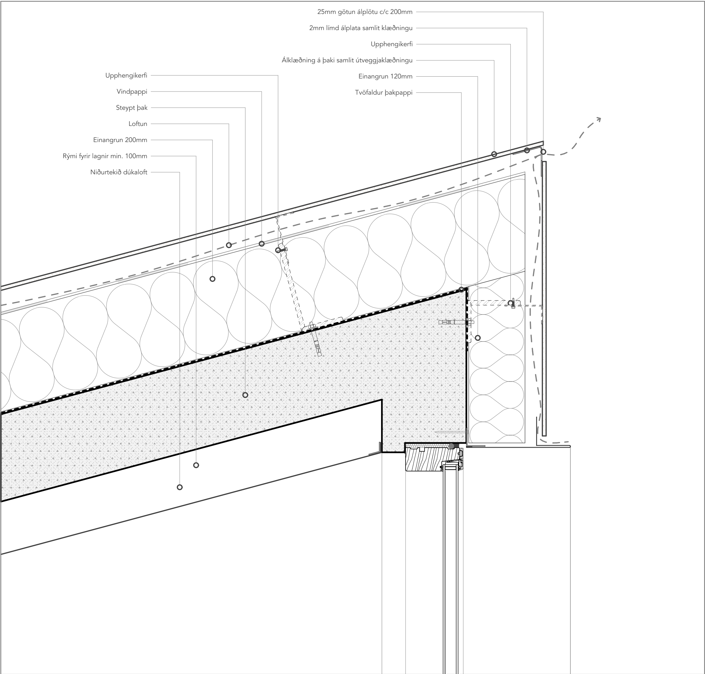
D-2 Einhalla þak - hæsti punktur 1:5
