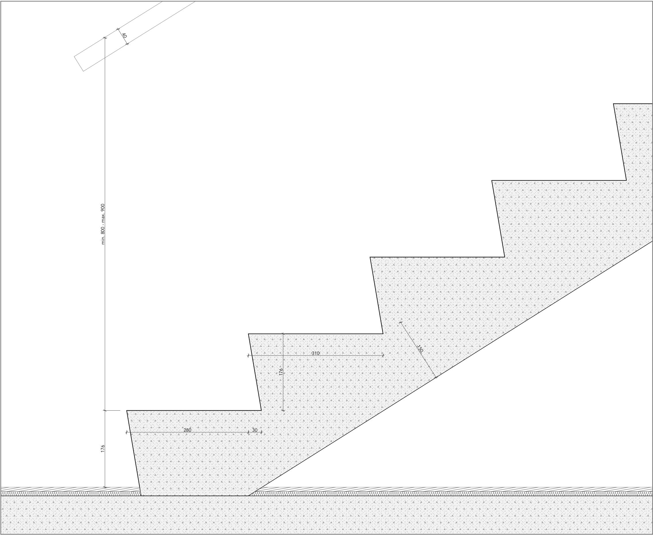
D-6 Stigateikning - Handlisti 1:5
