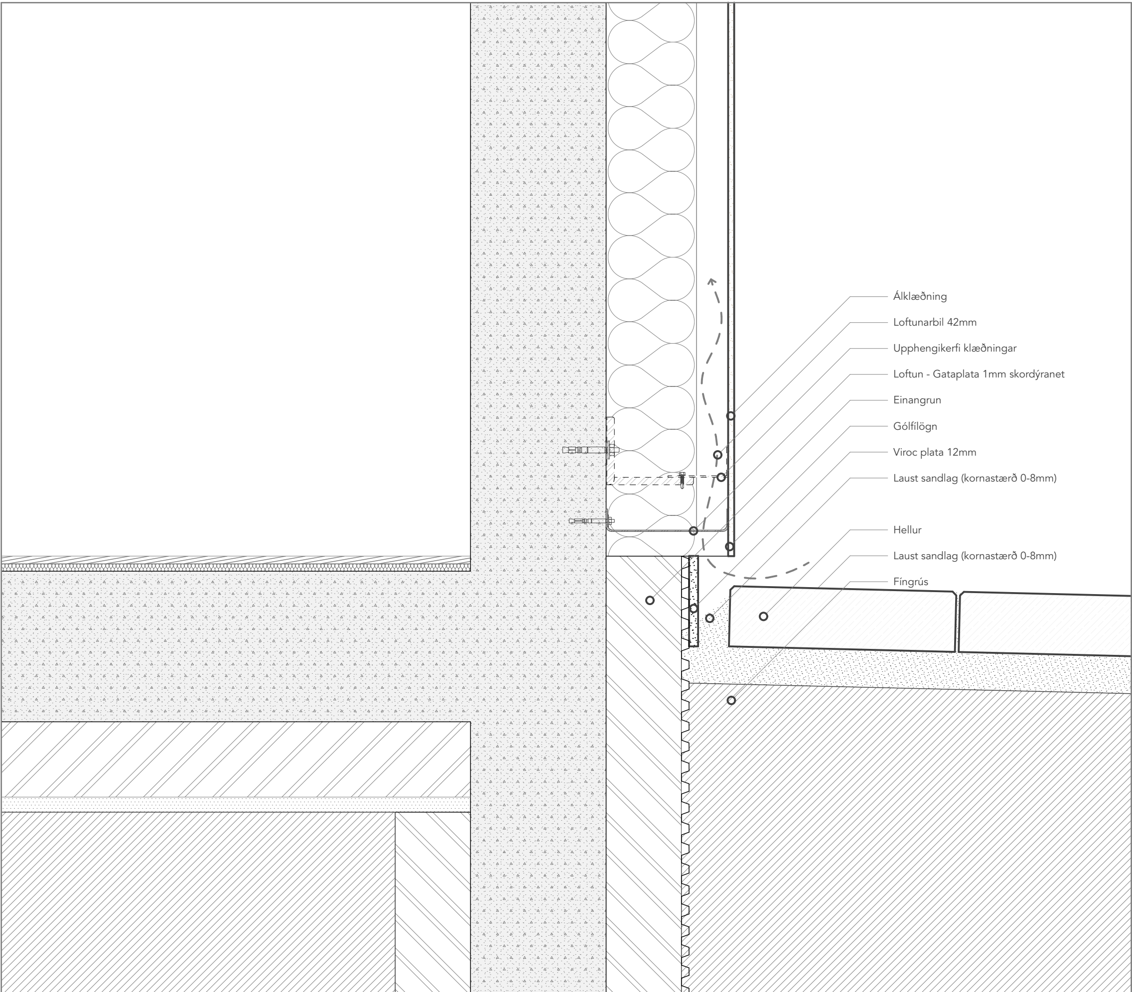
D-4 Útveggur við hellulögn 1:5
